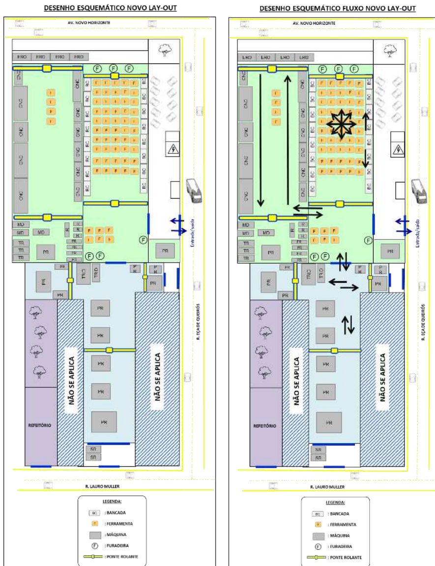
Figura 3: Perspectiva de do layout dos equipamentos no espaço A.1
